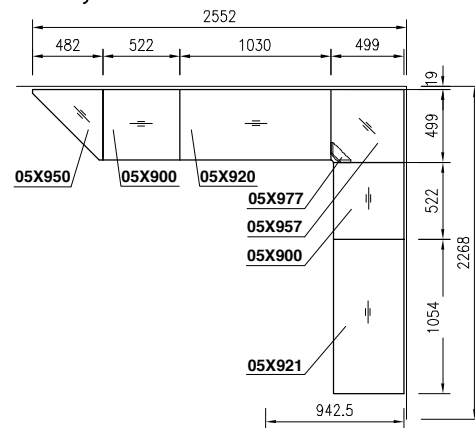
Půdorysná sestava 2
