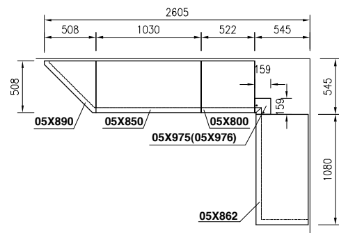
Půdorysná sestava 3
