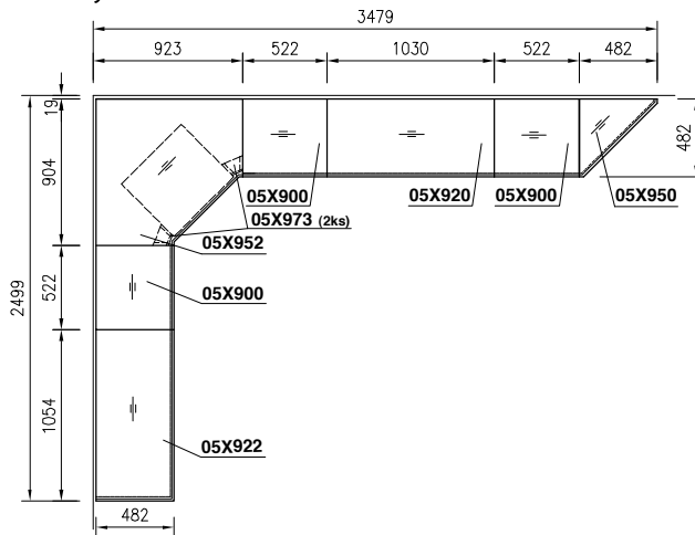
Půdorysná sestava 1
